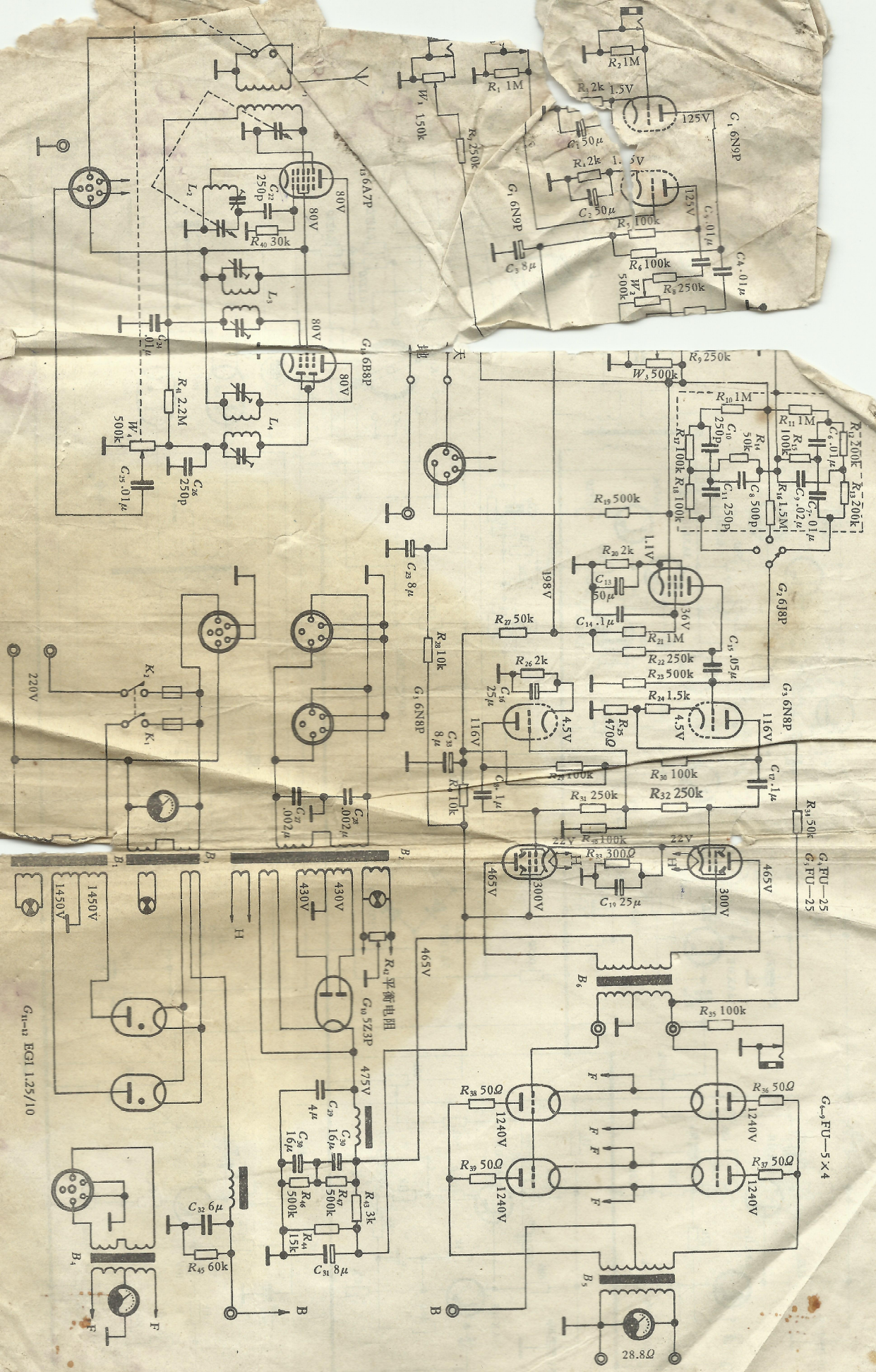
天津 500 瓦扩音机电路图
